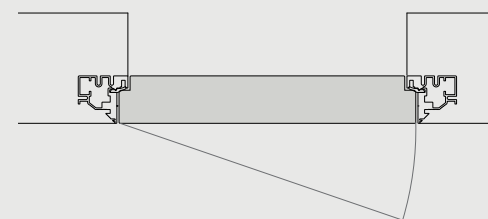
SEZIONE ORIZZONTALE PORTA A TIRARE SX Horizontal section door to pull left
