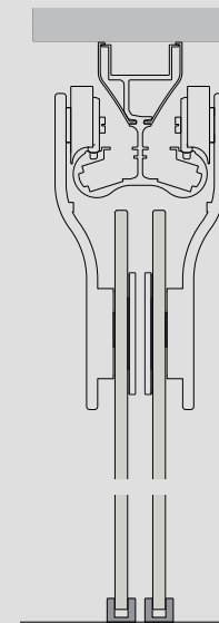
BINARIO A SOFFITTO A 2 VIE 2 ways ceiling rail
