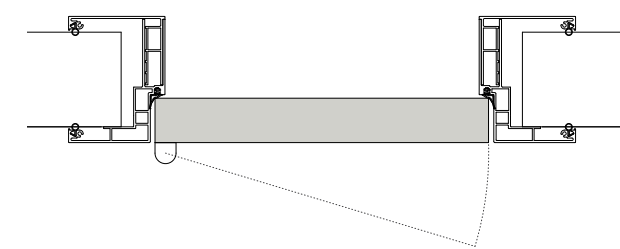
SEZIONE ORIZZONTALE PORTA A TIRARE CON STIPITI A 45° Horizontal section pull door with 45° jambs
