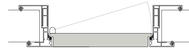
SEZIONE ORIZZONTALE PORTA A SPINGERE CON STIPITI A 45° Horizontal section door to push with 45° jambs
